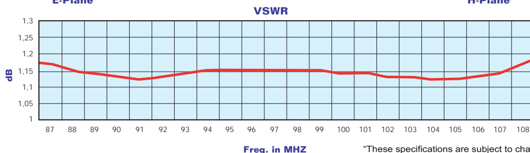
E-Plane
