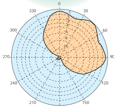
H-Plane
