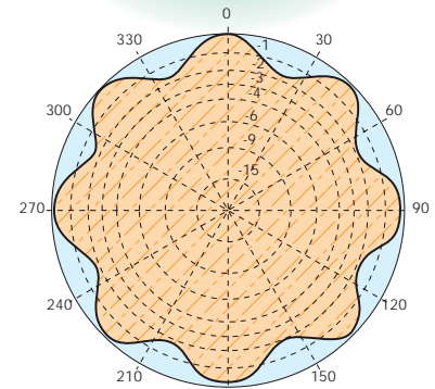
H-Plane
